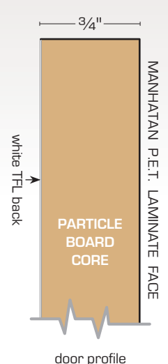
door profile
